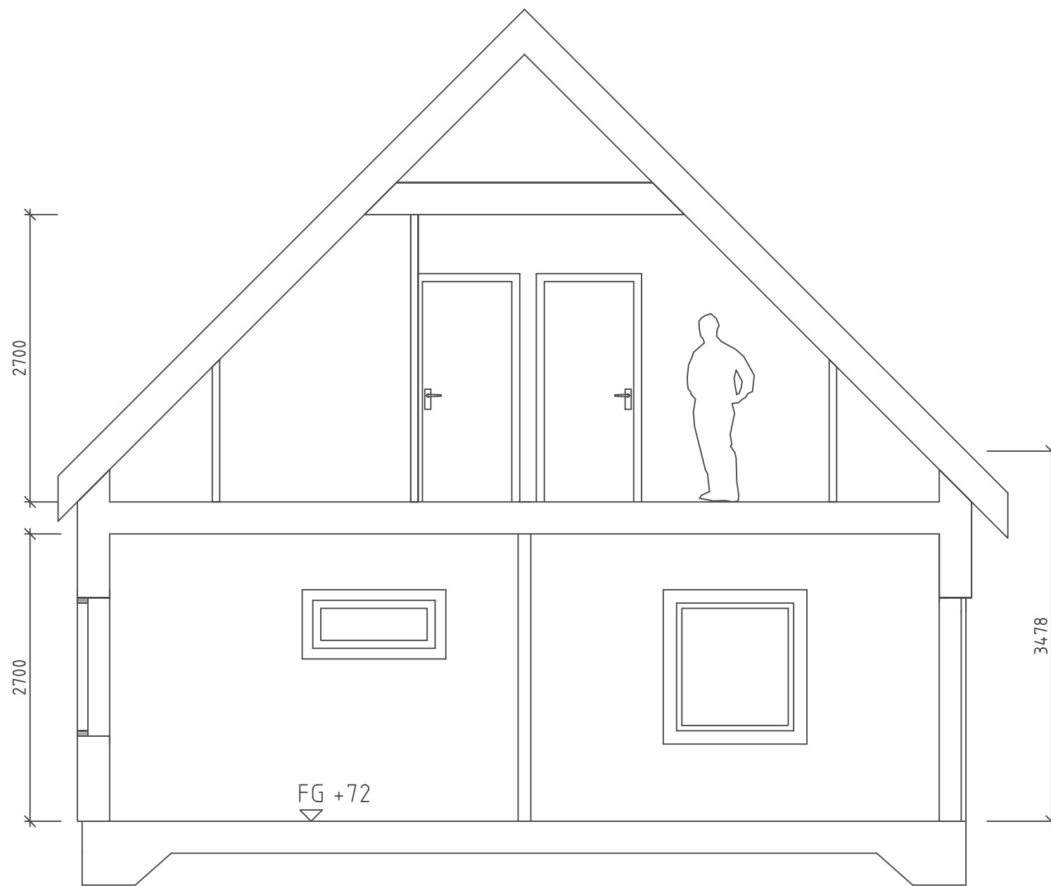
SEKTION A-A
